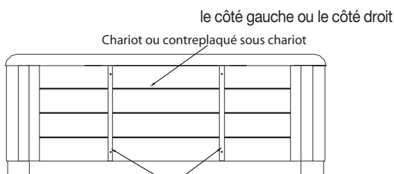
Longerons verticaux dissimulés du châssis du spa, espacés de 68,6 cm
